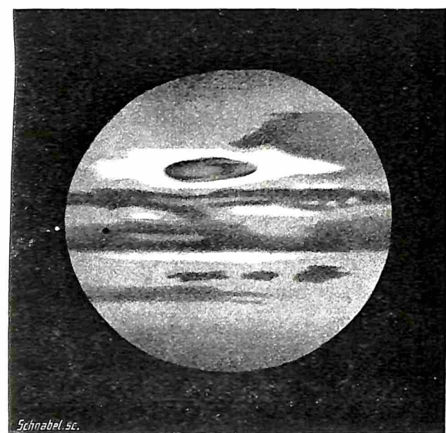
De satelliet is juist buiten den rand der schijf getreden; zijn schaduw is daarop nog zichtbaar.
